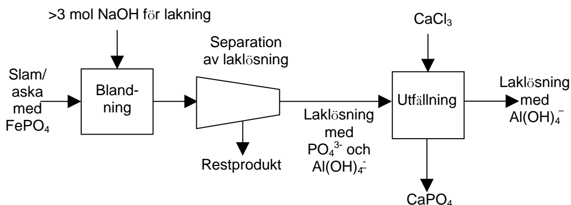
Figur 4. Lakning med bas följt med fällning av fosfat som kalciumfosfat.
